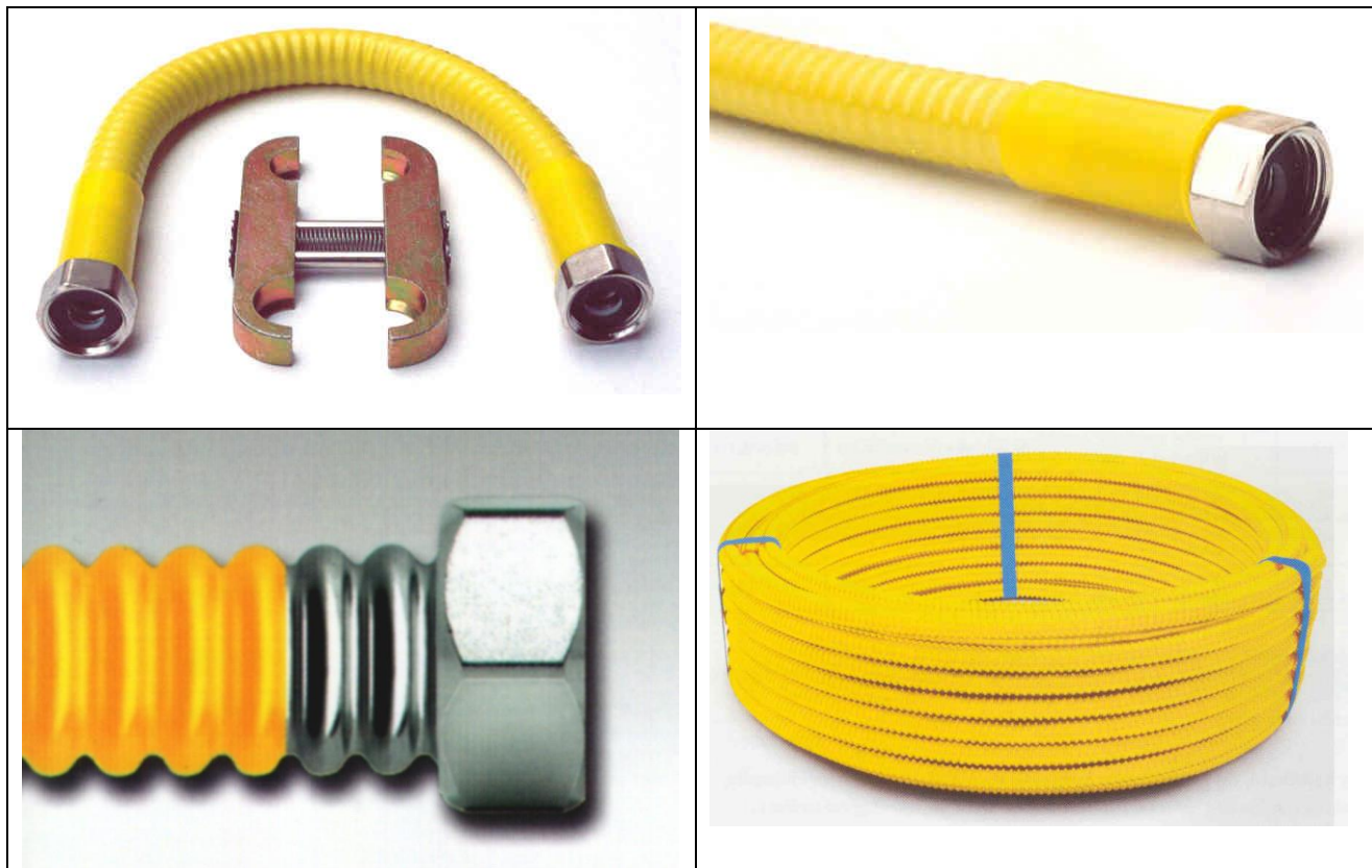
A GEBO SEE Kft. által forgalmazott Eurotis gyártmányú Variogas szerelvény
